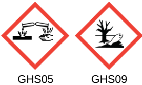
GHS05
